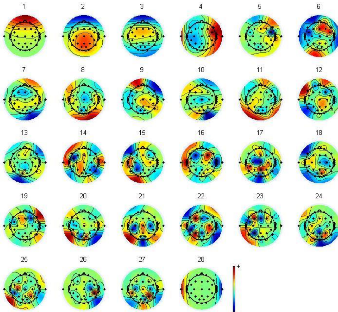
PCA version
